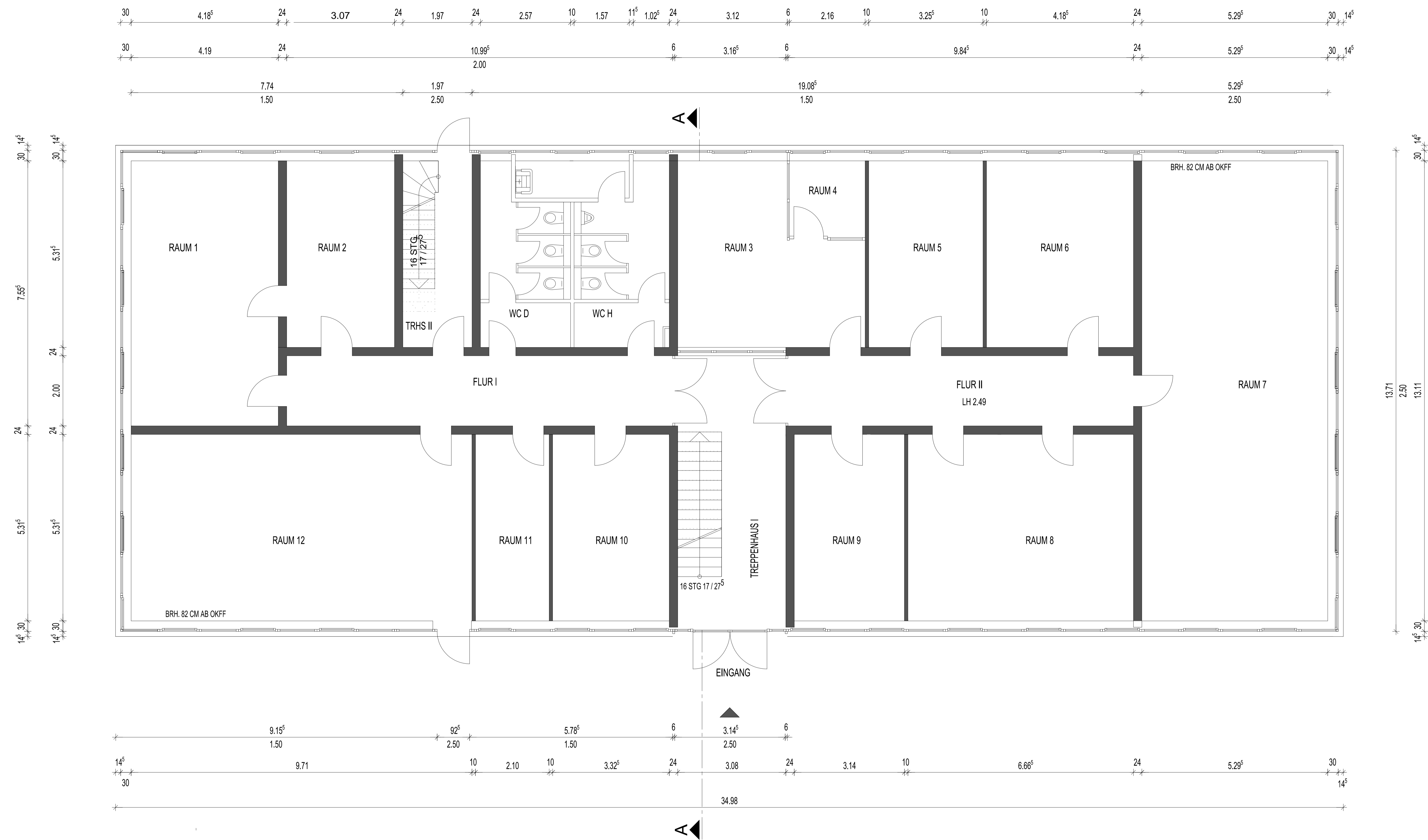
■ Grundriss Erdgeschoss
